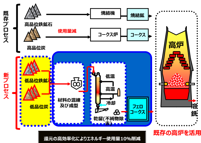
<フェロコックス技術の開発事業のイメージ>
