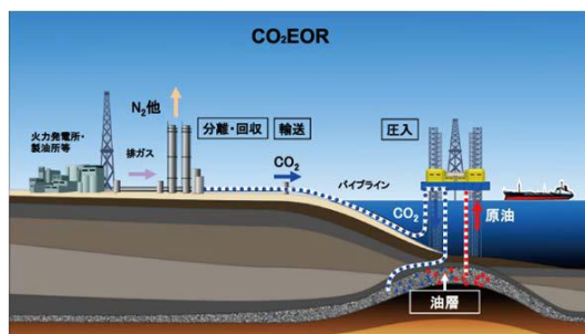
＜CO2-EOR＞
