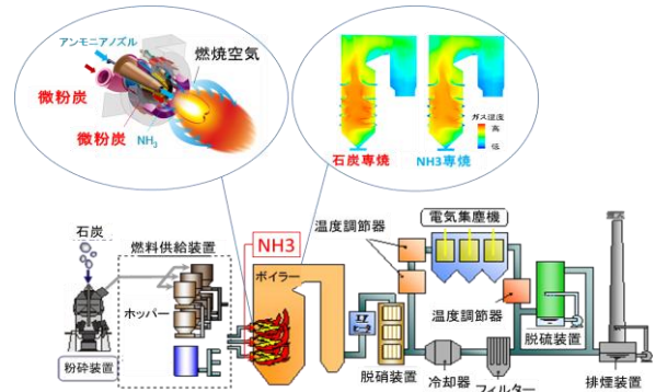
<アンモニア混焼>
